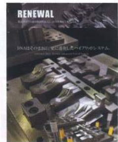
金属光造形複合加工機 EXCESS-HYBRIDII
