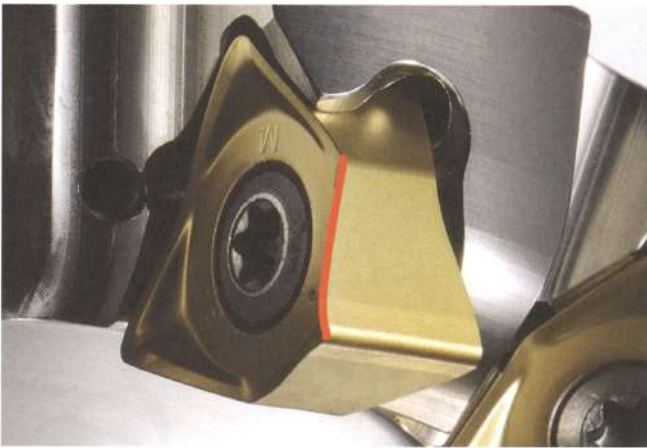
最適なすくい面の曲線切れ刃形状
