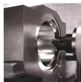
直角肩削り フライスカッター CoroMill® MS60
