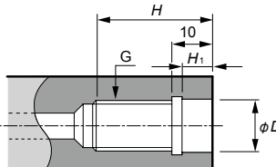
モジュラーミル 取付け部
