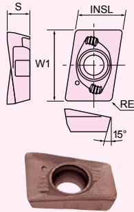
Fig.1 底刃用インサート Inserts on end
