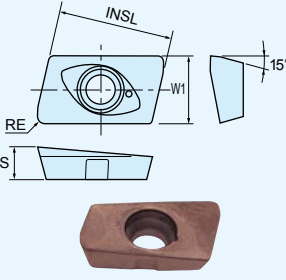
Fig.2 外周刃用インサート Inserts on periphery
