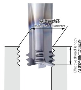
スレッドミルによる加工 Processing by thread mill
