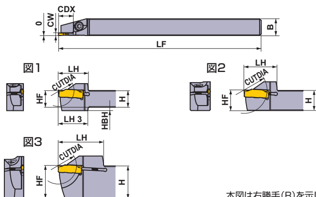
本図は右勝手(R)を示します。
