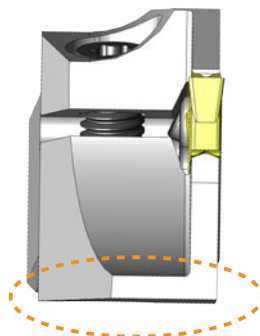
シミュレーション解析 変位量: 0.013
