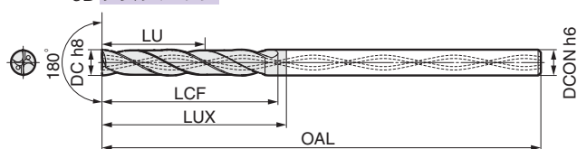
●5D ダブルマージン
