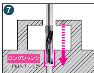
深位置への座ぐり加工
