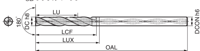
●3D シングルマージン
